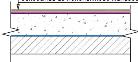
Сечение готового покрытия.
