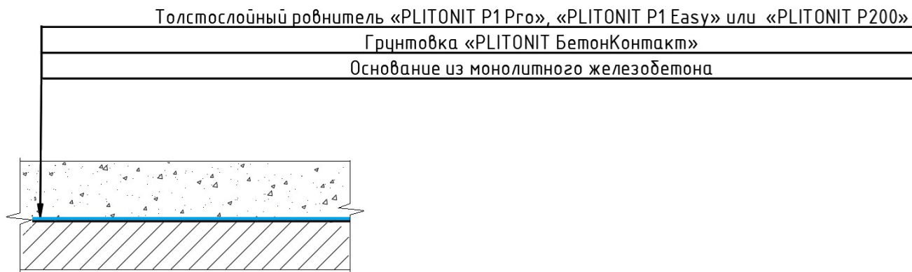
Сечение готового покрытия толстослойного ровнителя.
